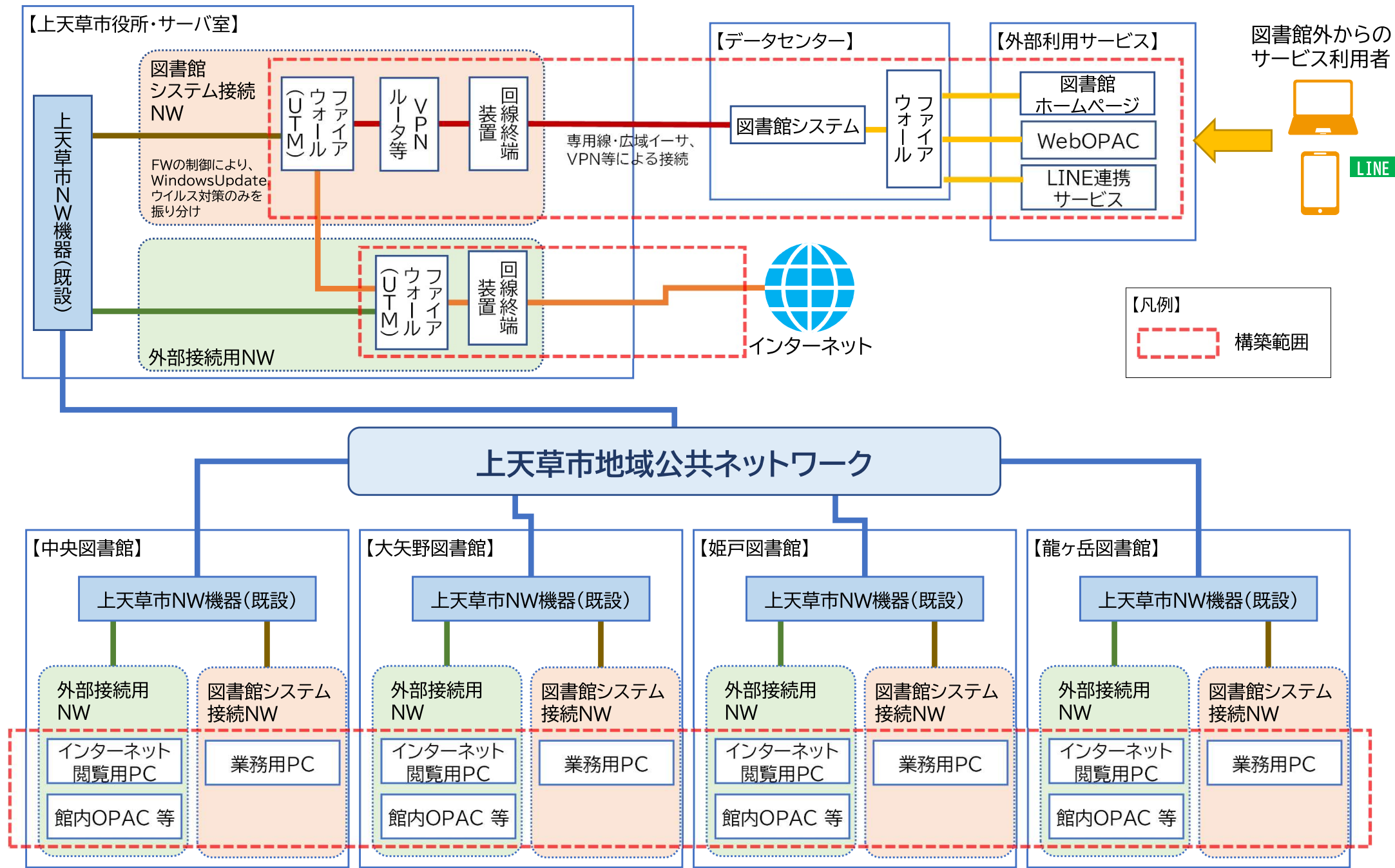
【全体構成図】
