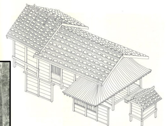
建物推定復元図
