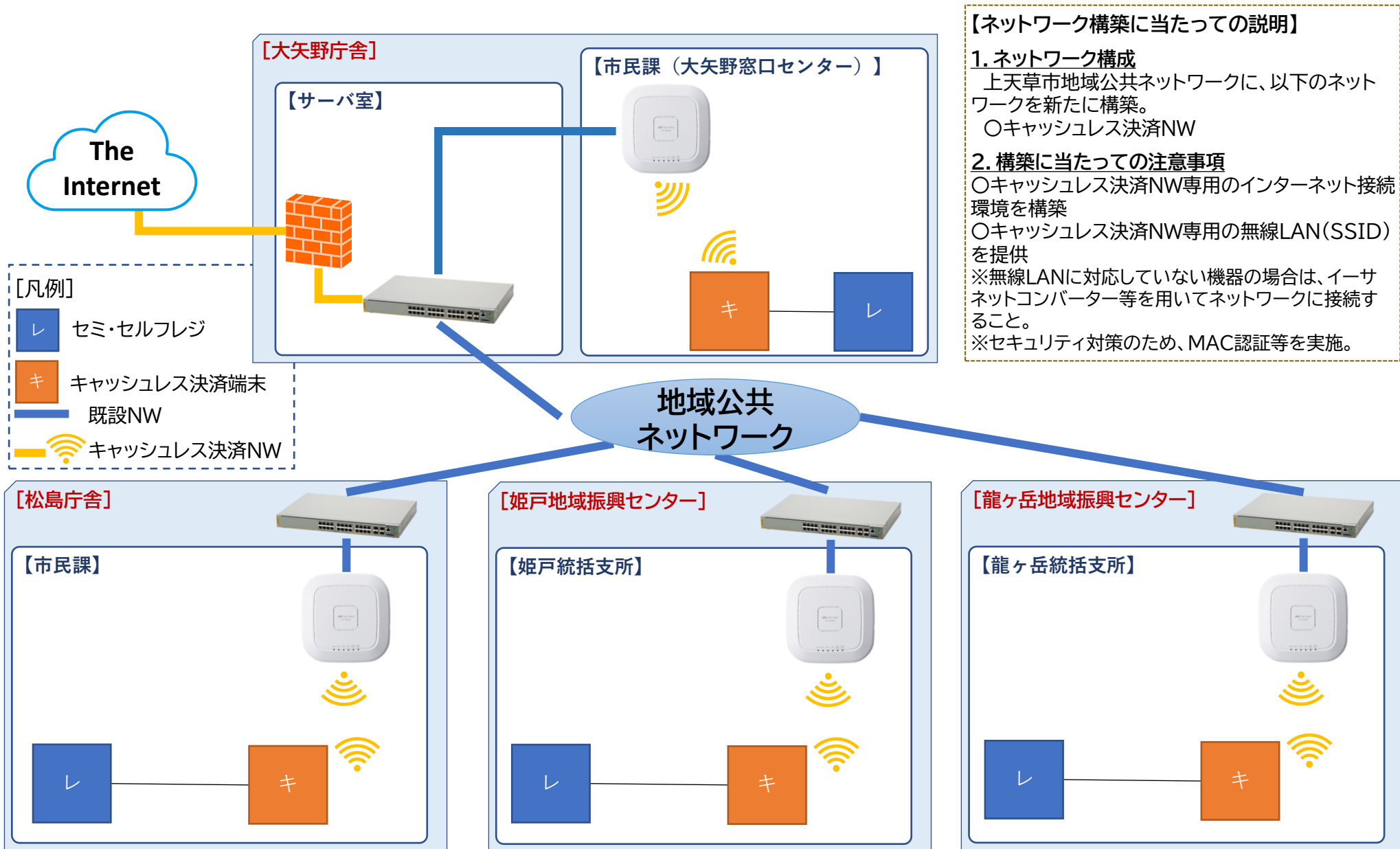
【ネットワーク構成図】
