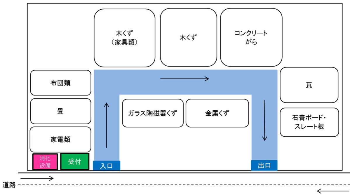
図3-2 二次仮置場の分別配置の例
