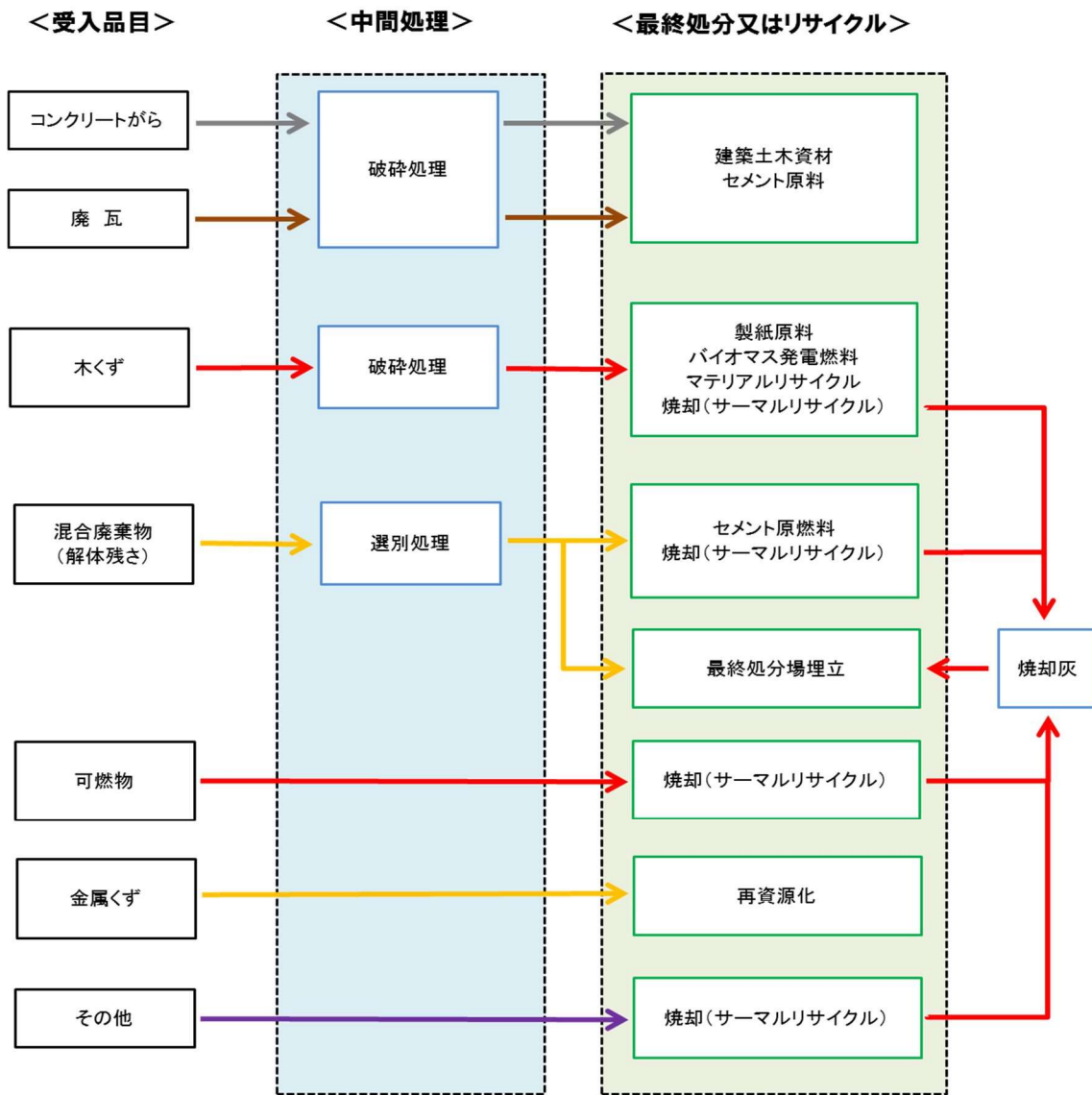
図 3-1 災害廃棄物処理フロー例
