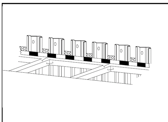
矢板及び腹起し設置間隔
