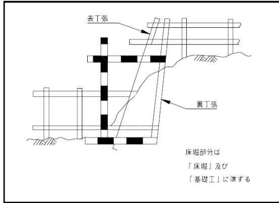
切取り法面
