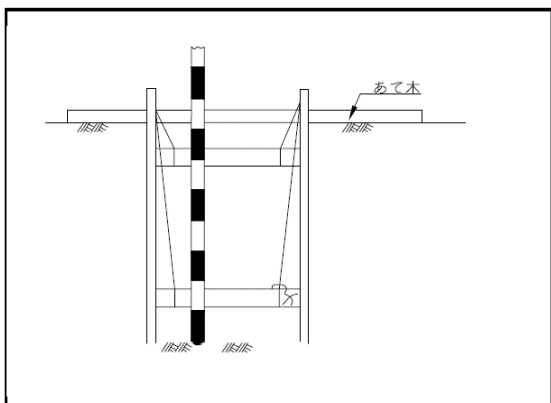
腹起し切梁の設置間隔
