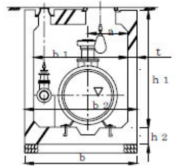
断面図（現場打）
