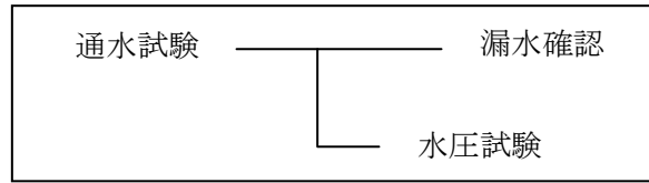
図－１ 通水試験の方法
