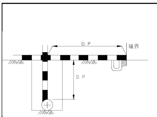
管布設位置
