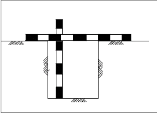
布掘り
