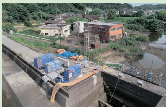
▲仮設ポンプ設置後の広崎排水機場
